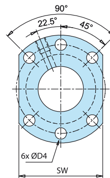
Bohrbild 1
